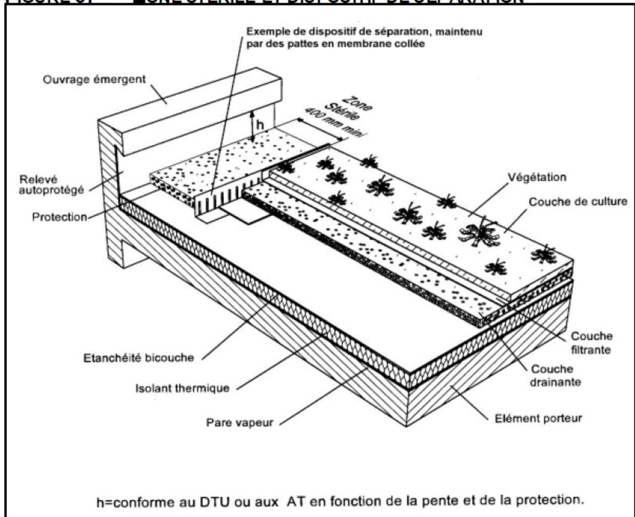
FIGURE 6: ZONE STERILE ET DISPOSITIF DE SEPARATION
